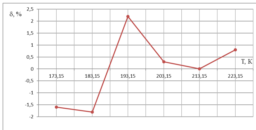
Рис. 2. График зависимости отклонения стандартных справочных данных от теоретических значений ( \delta_x = (X_{\text{ССД}} - X_{\text{расч}})/X_{\text{ССД}} где X соответственно \lambda_0 )
