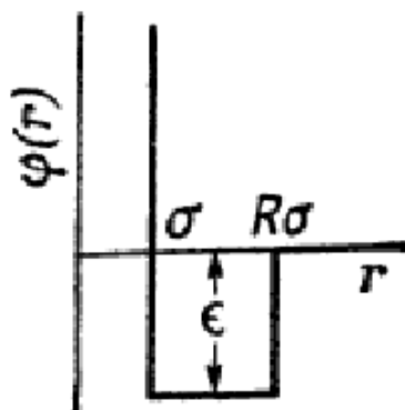
Рис 1. График потенциала прямоугольной ямы: \sigma - диаметр молекулы; \epsilon - глубина потенциальной ямы; R – расстояние между молекулами.
